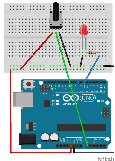
Breadboard oppkobling for eksempel 3
