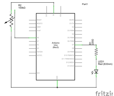
Koblingskjema for eksempel 2
