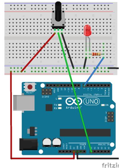
Breadboard oppkobling for eksempel 2
