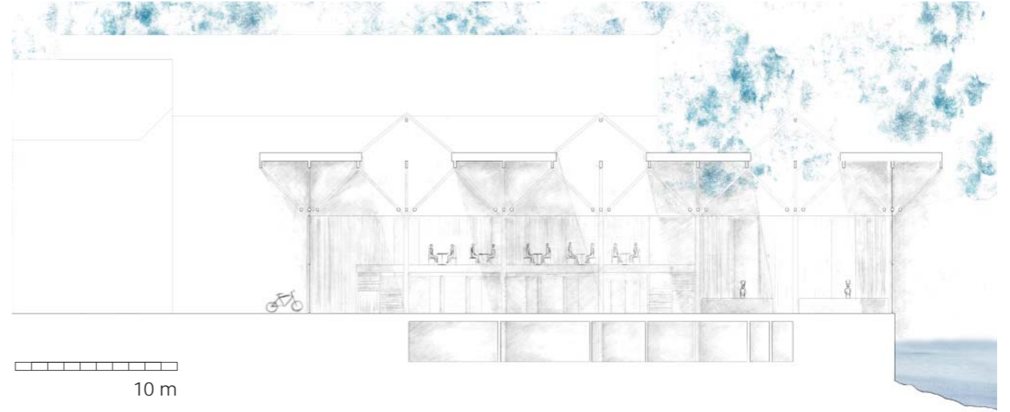
Snitt B-B'
