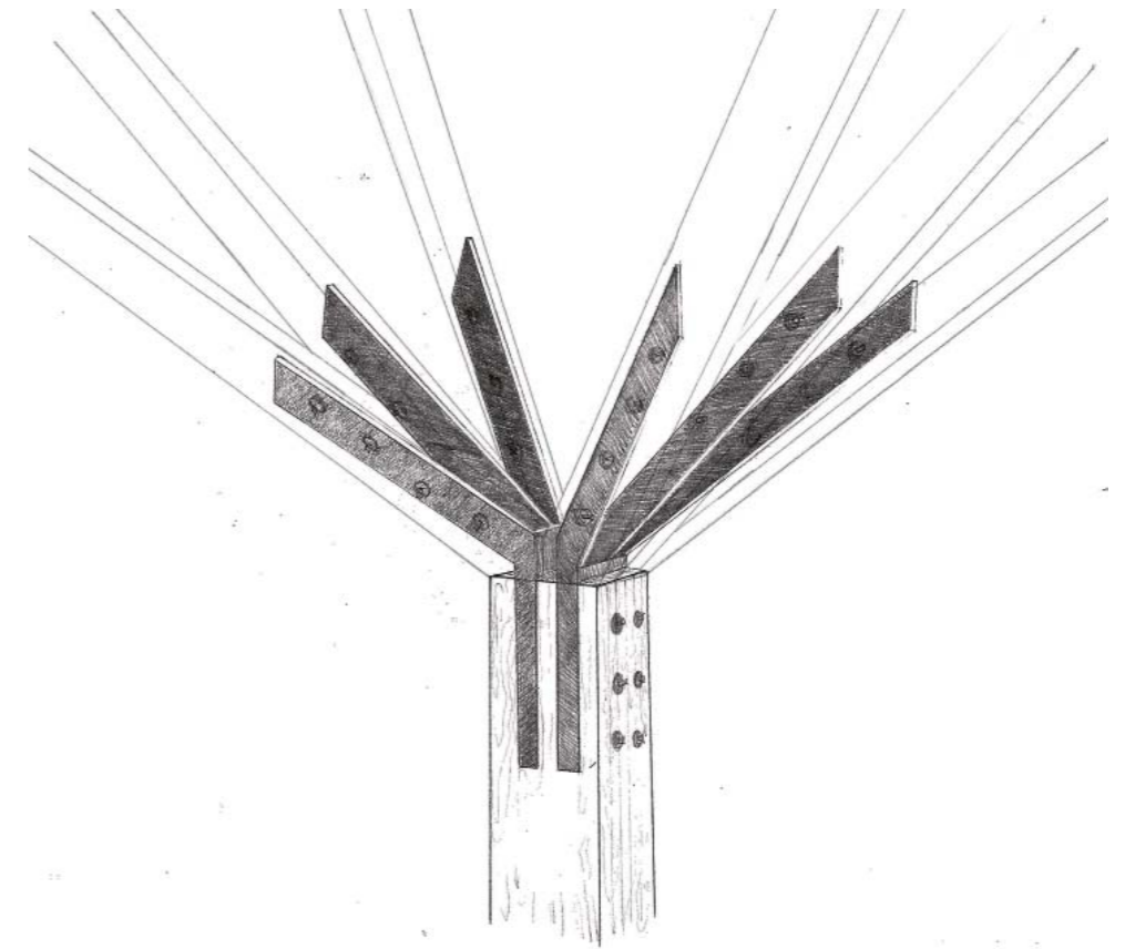
Prinsipp for takkonstruksjon
