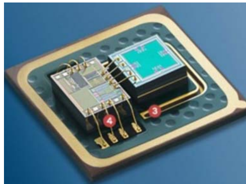
Figur 7.5 Trykksensoren består av en piezo-resistiv skive med elektroder (til høyre). Til venstre sees elektronikken.
