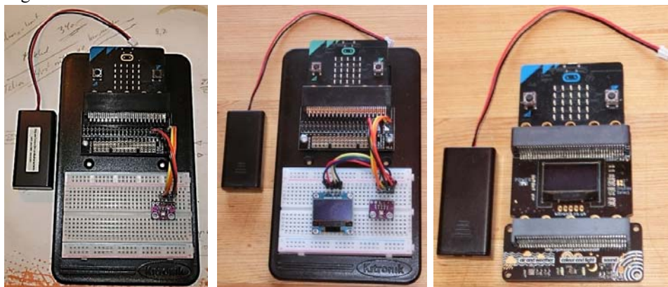
Figur 7.7 Oppkoblet prototyp av barometrisk høydemåler med micro:bit, lufttrykkssensor, display og batteri. A) bygget på prototypkort med BMP280 og uten OLED display. B) Som A), men med OLED-display. C) Bruker Enviro:bits trykksensor og Kitroniks OLED-display (SSD1306).
