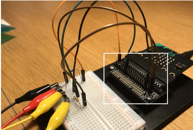
220Ohm (rød-rød-brun)
