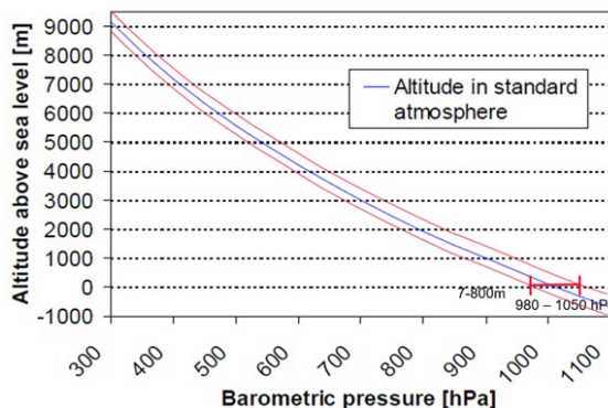
Figur 7.2 Beregnet høyde over havnivået som funksjon av lufttrykk. Det er indikert hvordan en ukalibrert måling vil kunne gi avvik på flere hundre høydemeter ved lavtrykk og høytrykk.
