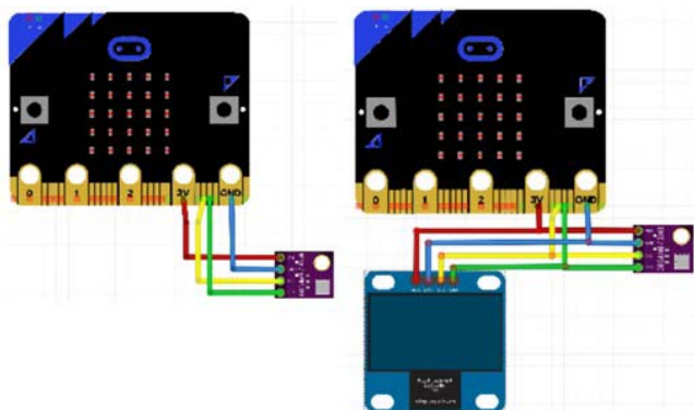
Figur 7.6 Til venstre, enklest mulig oppkobling med kun BMP280. Til høyre, høydemåler supplert med et bedre display (SSD1306) enn det innebygde LED-displayet til micro:bit.
