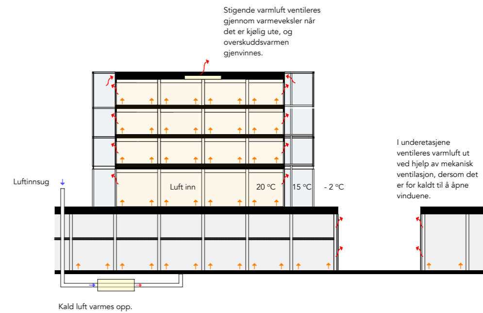
Ventilasjonsprinsipp vinter
