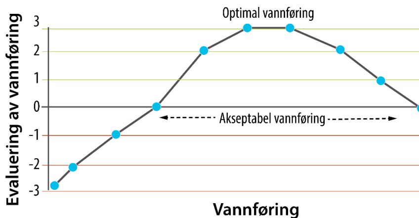
Figur 5. 'Flow-curve' som illustrerer ikke-akseptabelt, akseptabelt og optimalt vannføringsnivå basert på brukerundersøkelser i 'The Structural Norm Approach' (Whittaker & Shelby 2002). Med tillatelse.
