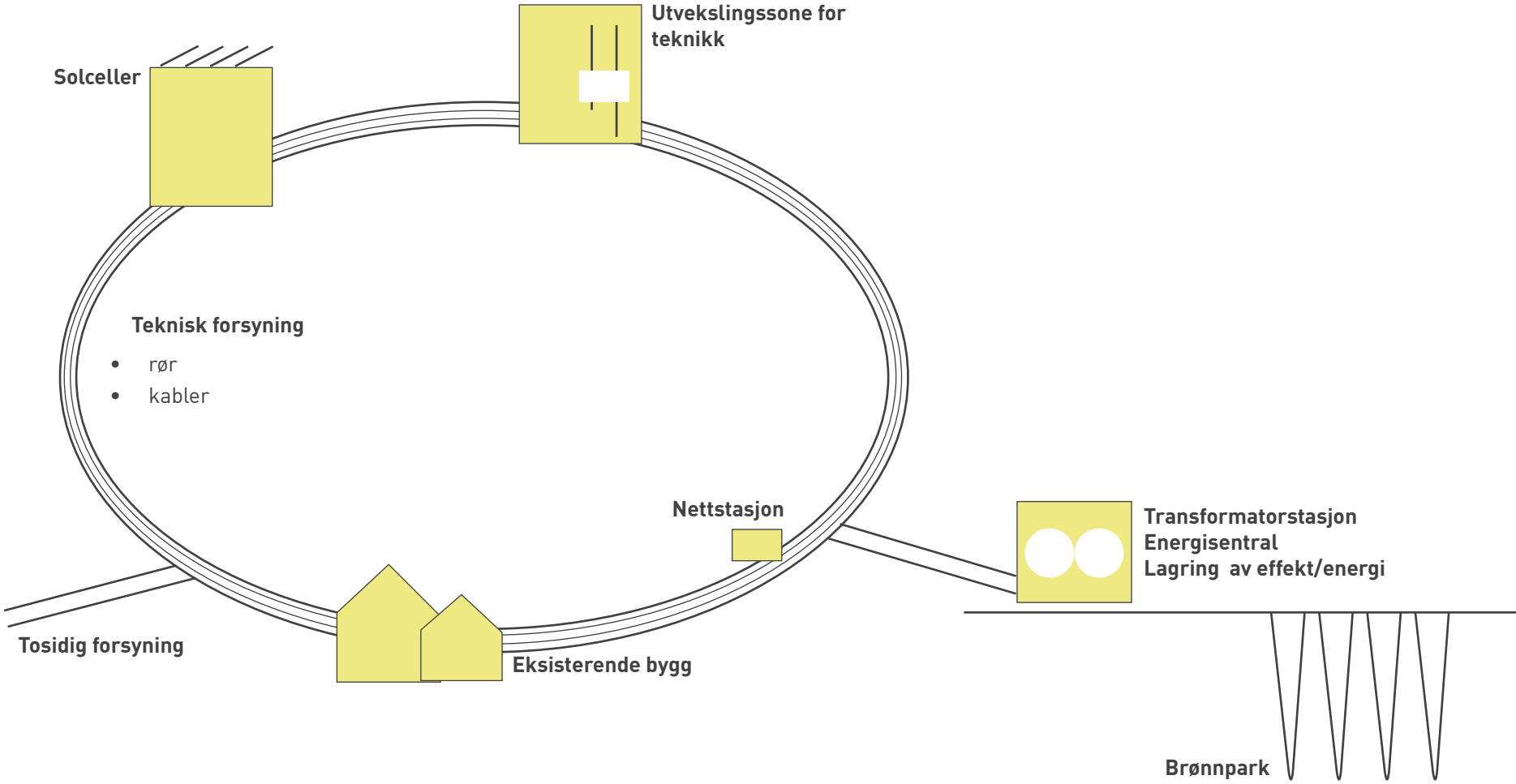
Figur 4. Ringstruktur for utveksling av energi og effekt, samt forsyningssikkerhet. En slik ringstruktur binder sammen bygg, områder, energiproduksjon og energilagring. Dette gjør at man kan ta vare på overskuddsenergi og unngå effekttopper.
