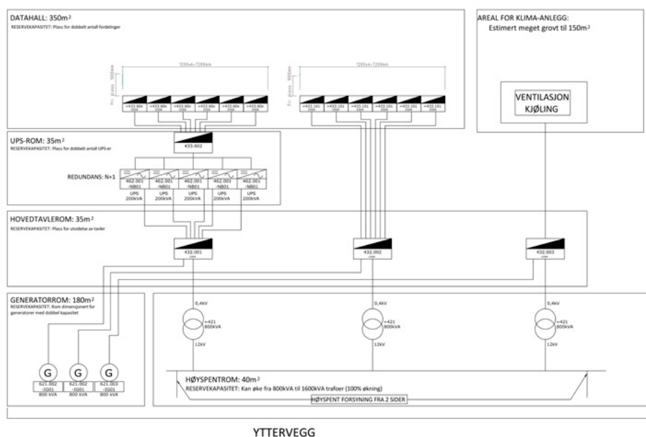
Prinsipp struktur for strømforsyning til datahall
