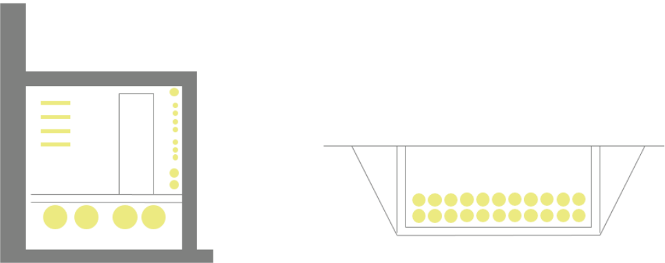
Figur 6. Eksempel på føringsveier i kulvert og nedgravd i støpt kanal.
