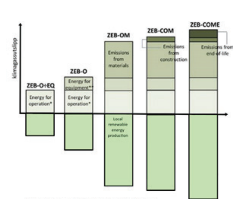
Figur 3. Ulike nivåer av ZEB-definisjoner. Grønne søyler under akse viser at lokal fornybar energiproduksjon minst må veie opp for det utslippet bygget generer.
