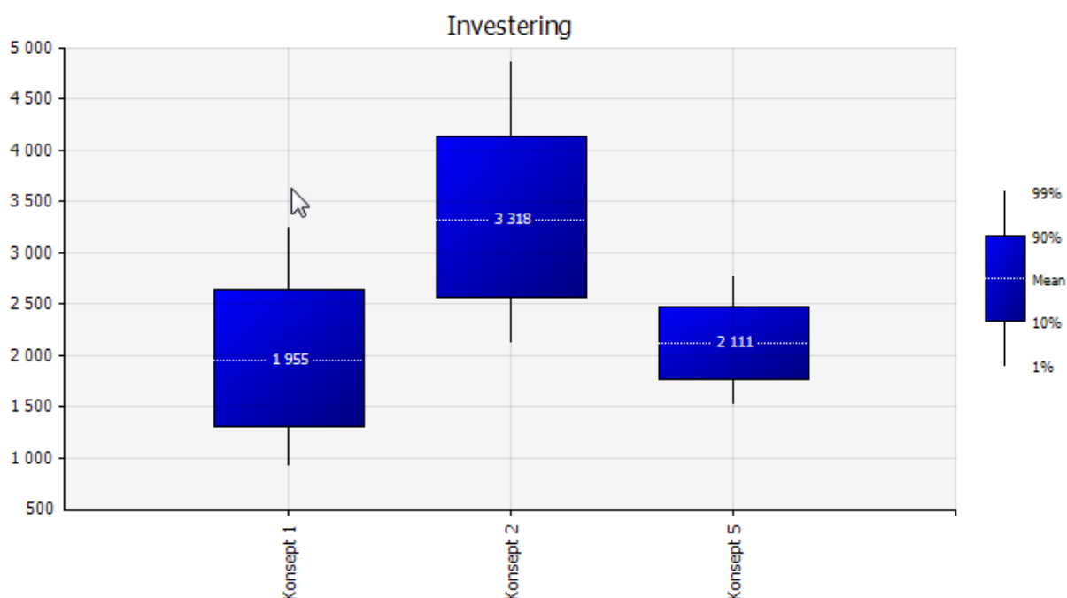
Figur 15: Box-plot med investeringskostnader for konseptene (MNOK)
