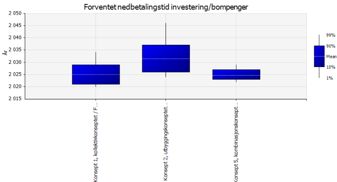
Figur 6: Forventet nedbetalingsår av investering, finansiert av bompenger
