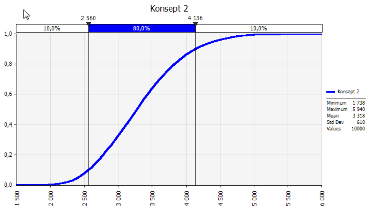
Figur 10: S-kurve Konsept 2 (MNOK)
