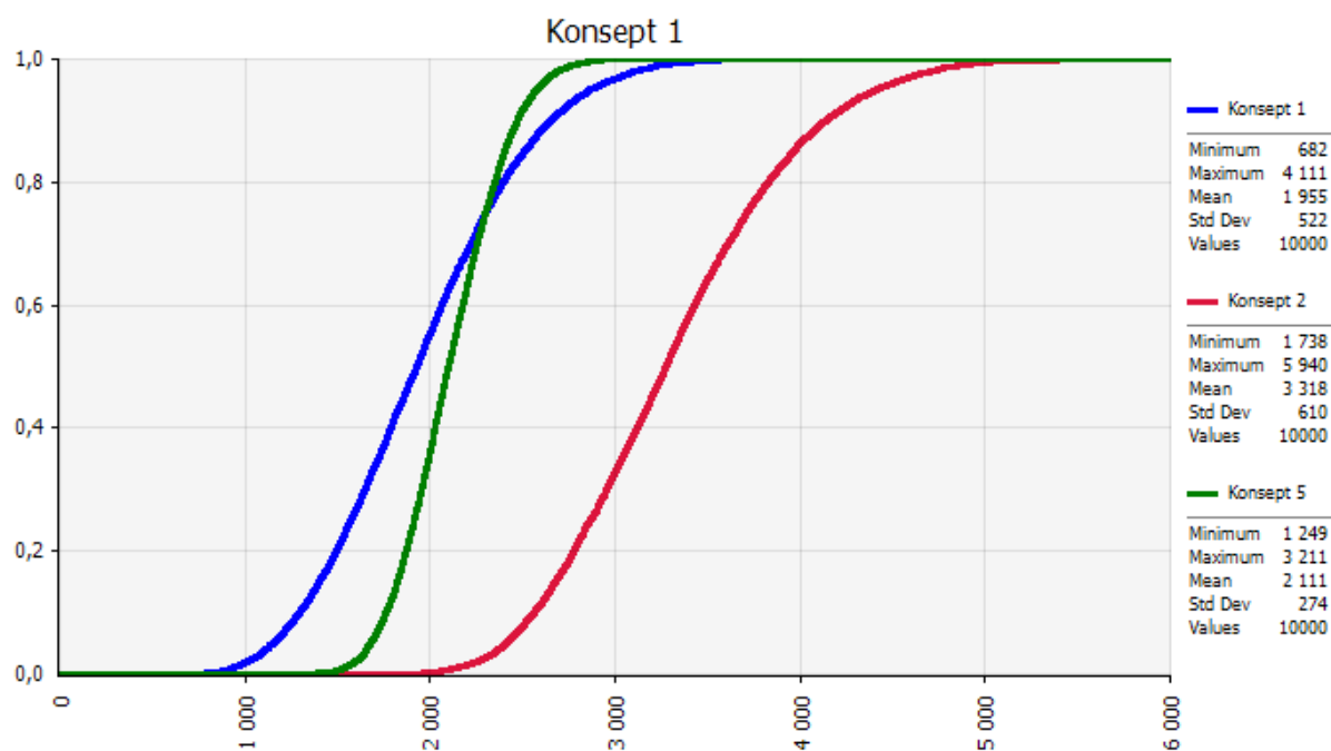
Figur 14: S-kurver med investeringskostnader for konseptene (MNOK)
