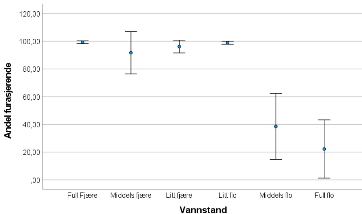
Figur 3.25. Gjennomsnittlig andel (prosent) furasjerende vadefugler ( \pm 2SE ) ved 15 totaltellingene ved ulike vannstander i sonene 1-3 fra midten av juli til slutten av oktober (uke 29-43) 2022. Andelen er beregnet slik at alle de 15 registreringene har lik innflytelse på gjennomsnittsverdien (se Kapittel 2.5). Det er summen av sonene 1-3 som er brukt.
