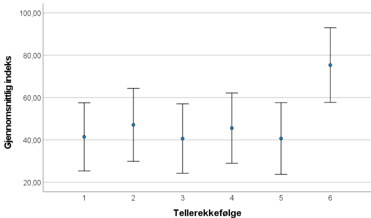
Figur 3.29. Gjennomsnittlig relative antall vadefugler ( \pm 2SE ) i forhold til tellerekkefølge ved 15 totaltellingene i sonene 1-3 fra midten av juli til slutten av oktober (uke 29-43). Indeksen er forklart i Kapittel 2.4, og gjør at alle de 15 registreringene har lik innflytelse på gjennomsnittsverdien. Det er summen av antall individer i sonene 1-3 som er brukt.
