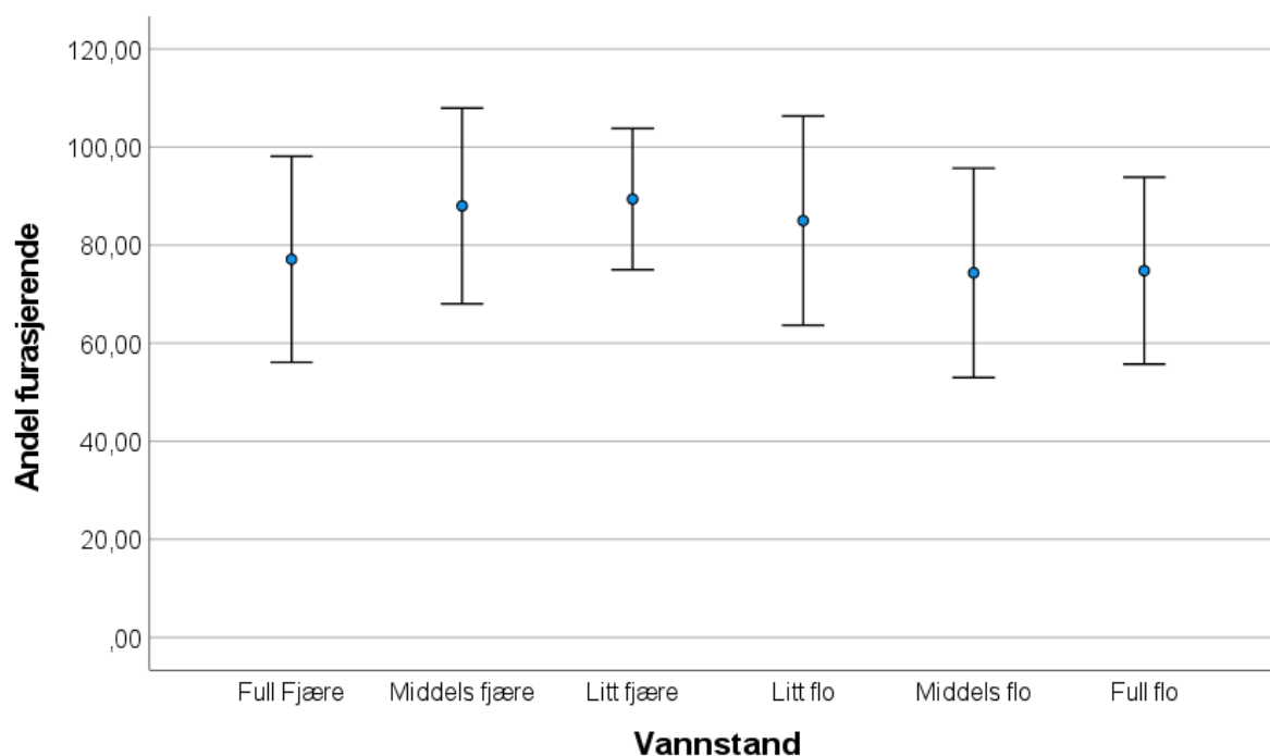
Figur 3.24. Gjennomsnittlig andel (prosent) furasjerende dykkender ( \pm 2SE ) ved 15 totaltellingene ved ulike vannstander i sonene 1-3 fra midten av juli til slutten av oktober (uke 29-43) 2022. Andelen er beregnet slik at alle de 15 registreringene har lik innflytelse på gjennomsnittsverdien (se Kapittel 2.5). Det er summen av sonene 1-3 som er brukt.
