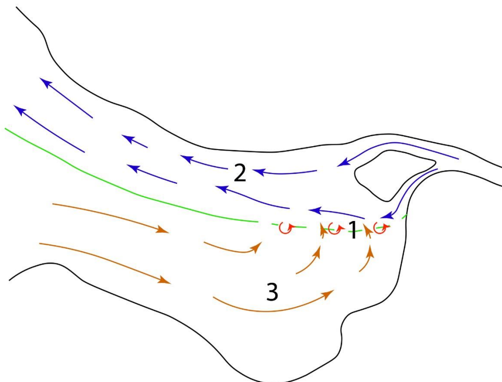
Figur 10. Skjematisk fremstilling av de dynamiske prosessene ved utløpet av Gaula. Når elva renner ut i fjorden blir det sterk turbulens ved fronten mellom ellevann og sjøvann (1). Denne turbulensen bidrar til å blande sjøvann inn i ellevannet. Strømmen av ellevann og medrevet sjøvann strømmer utover fjorden på høyre side grunnet Coriolis-kraften (2). Sjøvannet som blir revet med av ellevannet må erstattes og dermed får vi kompensasjonsstrøm (3).
