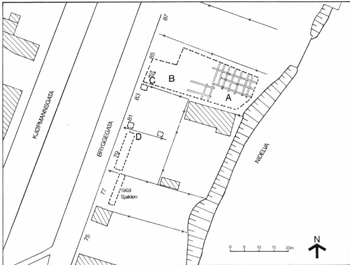
Figur 1. Plan over utgravningen i Kjøpmannsgata 75-85, med avmerking av område A, B, C og D
