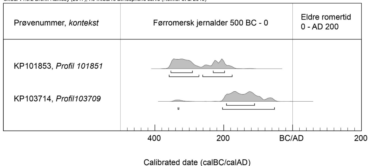
Figur 7: Dateringskurve over daterte ^{14}\text{C} -prøver fra kulturlag 102240. Jf. tabell 7.
