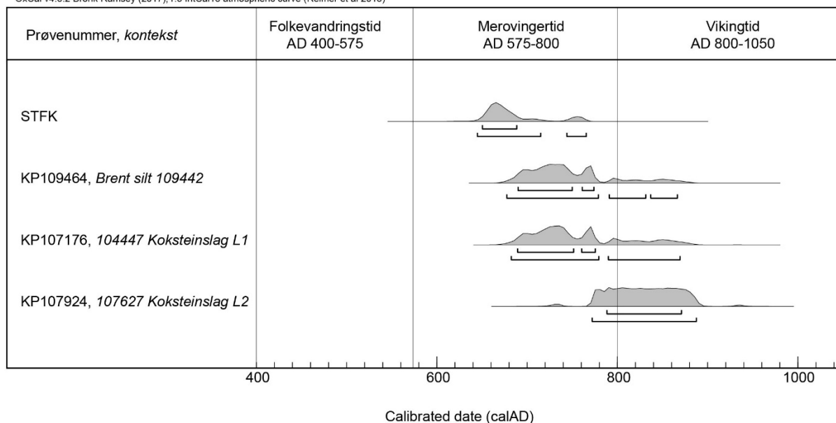
Figur 14: Dateringskurve over daterte ^{14}\text{C} -prøver fra koksteinslaget. Jf. tabell 8.
