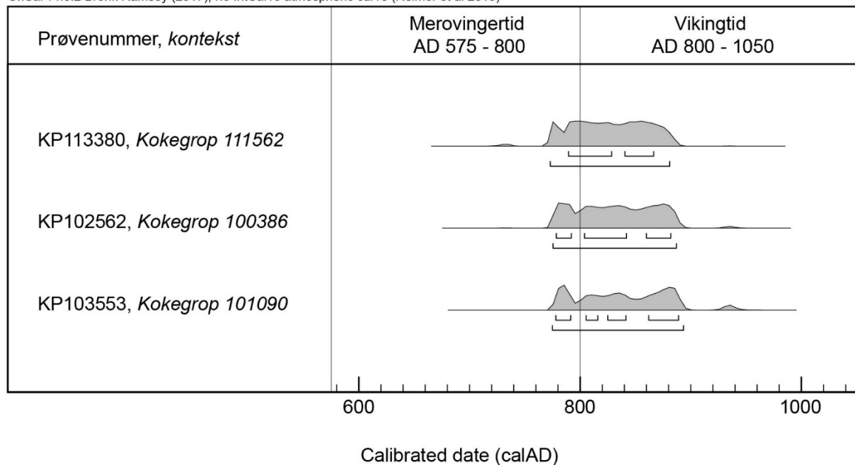
Figur 19: Dateringskurve over øvrige daterte 14 C-prøver fra kokegroper som ikke lå i koksteinslaget. Jf. tabell 10.
