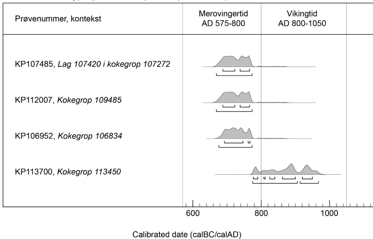
Figur 18: Dateringskurve over daterte 14 C-prøver fra kokegroper som lå i koksteinslaget. Jf. tabell 9.
