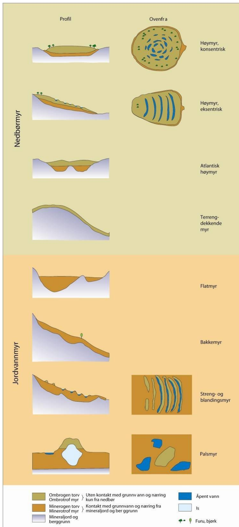
Figur 1. Skjematisk framstilling av noen hovedtyper av myr (myrmasivtyper). Fra Moen (1998).
