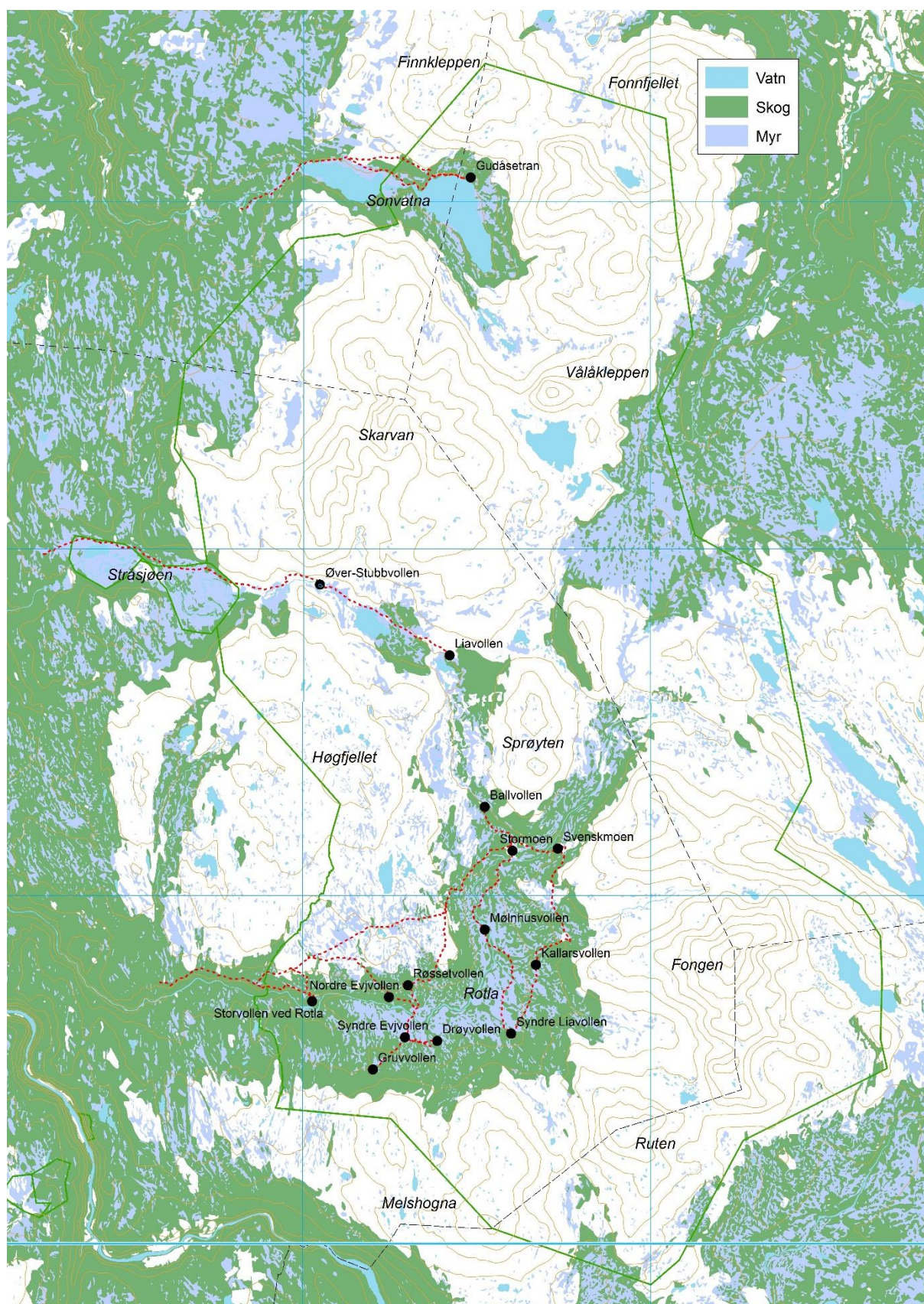
Figur 1. 15 setervoller kartlagt og vurdert som naturtypelokaliteter i 2014-2015 i Skarvan og Roltdalen nasjonalpark. Kartleggingsruter er vist med røde, stipla linjer, verneområder med grønne linjer. 10 x 10 km rutenett er i format UTM WGS84 , sonebelte 32 V og 100 km-rute PR. FKB-grunnlagsdata er brukt med tillatelse fra Norge digitalt.
