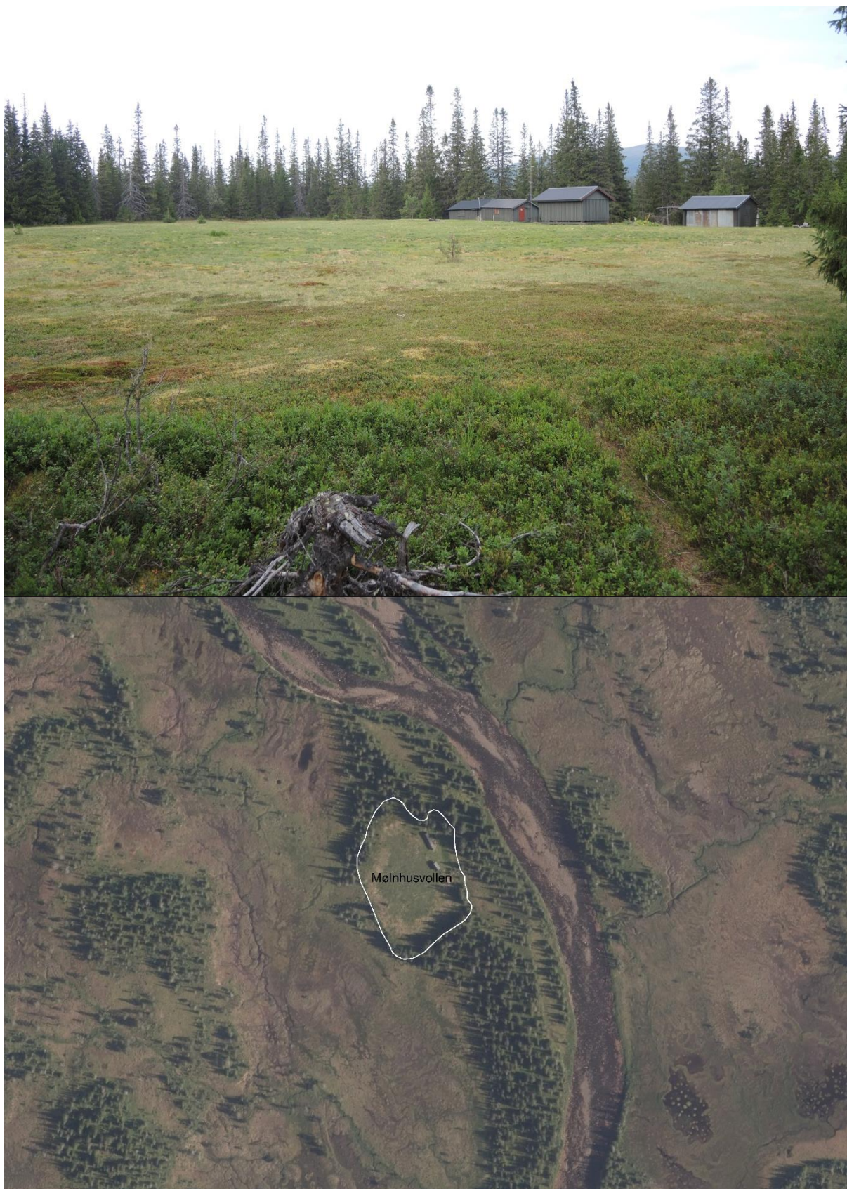
Figur 8. Mølnhusvollen sett fra sør mot nord, vollen har nylig blitt rydda (antakelig med beitepusser). Foto Anders Lyngstad 25.8. 2015. Kartutsnitt (ca. 700 x 500 m) er orientert nord-sør, ortofoto (opptak 22.7. 2014) er brukt med tillatelse fra Norge digitalt.
