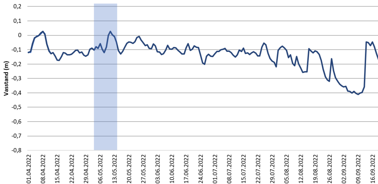
Figur 5. Eksempel på variasjon i vasstand gjennom sesongen 2022 på Sølendet. Data frå prøveflate 2F som har vore uslått i over 70 år. Det meste av snøen smelta i perioden 4.-14. mai (blå skravur).
