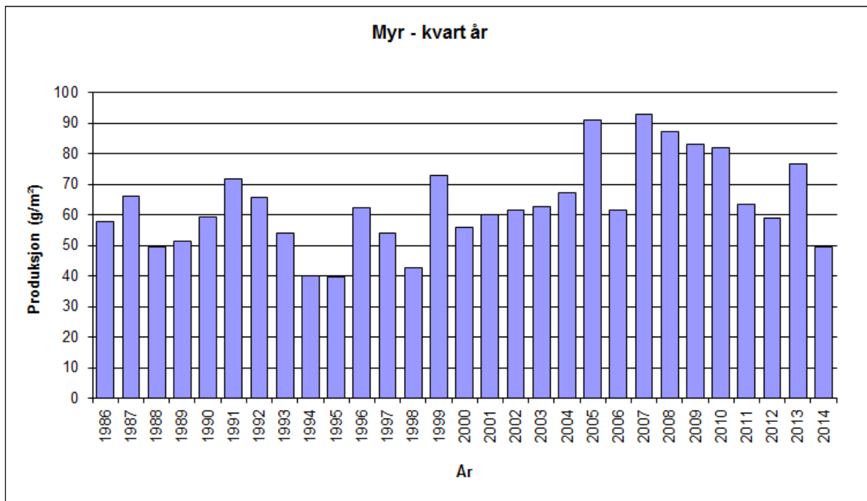
Figur 2. Gjennomsnittleg produksjon i rikmyrsamfunn på Sølendet i perioden 1986-2014. Resultat frå prøveflater på rikmyr som er slått med lå kvart år sidan slutten av 1970-talet.
