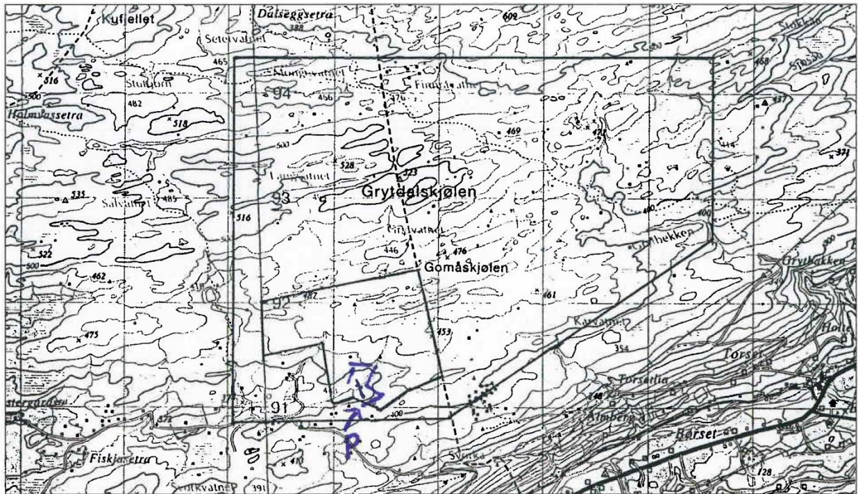
Figur 1. Kart over Tågdalen naturreservat (markert strek) med nærmeste omgivelser. Fra kartblad M711, 1421 II. NQ 00-08, 90-05 med rutenett 1 km 2 . P: parkeringsplass. Blå strek: natursti
