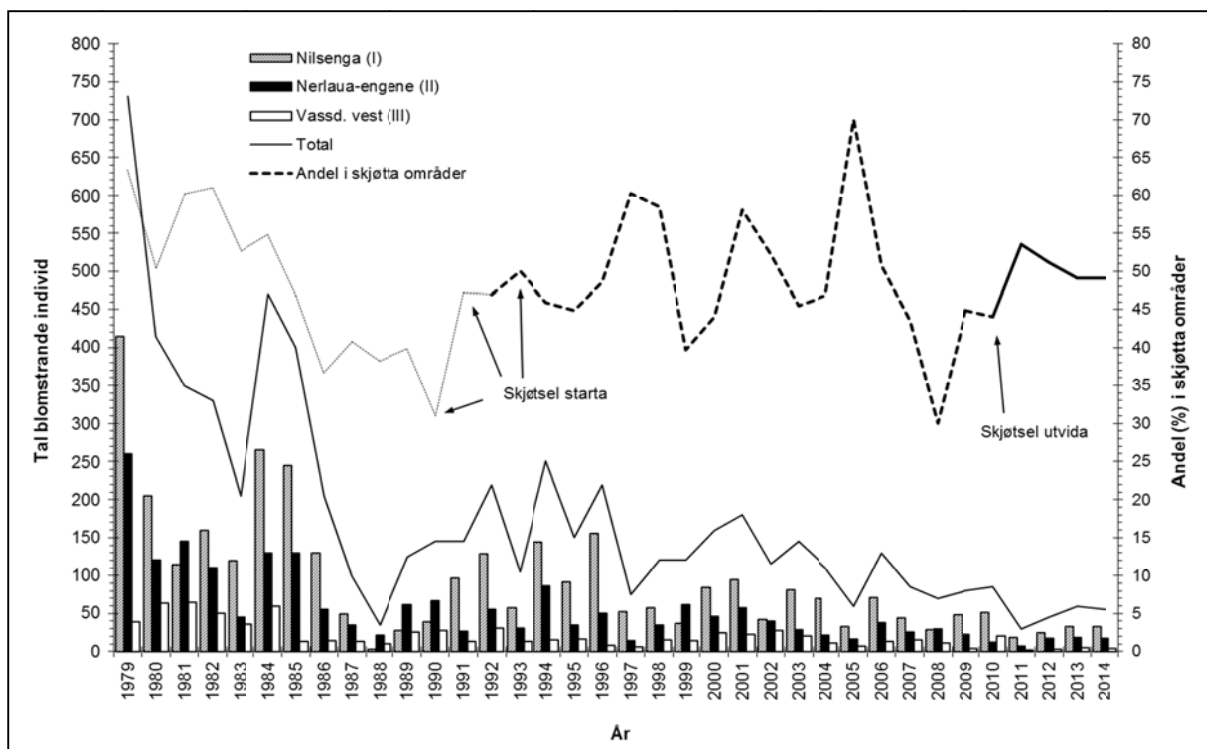
Figur 1. Blomstring av svartkurle ( Nigritella nigra ) i Sølandet naturreservat. Figuren viser talet på blomstrande individ innanfor reservatgrensene, og delen av det totale talet på blomstrande individ som finst på dei areala som no er skjøtta (tjukk stipla linje).
