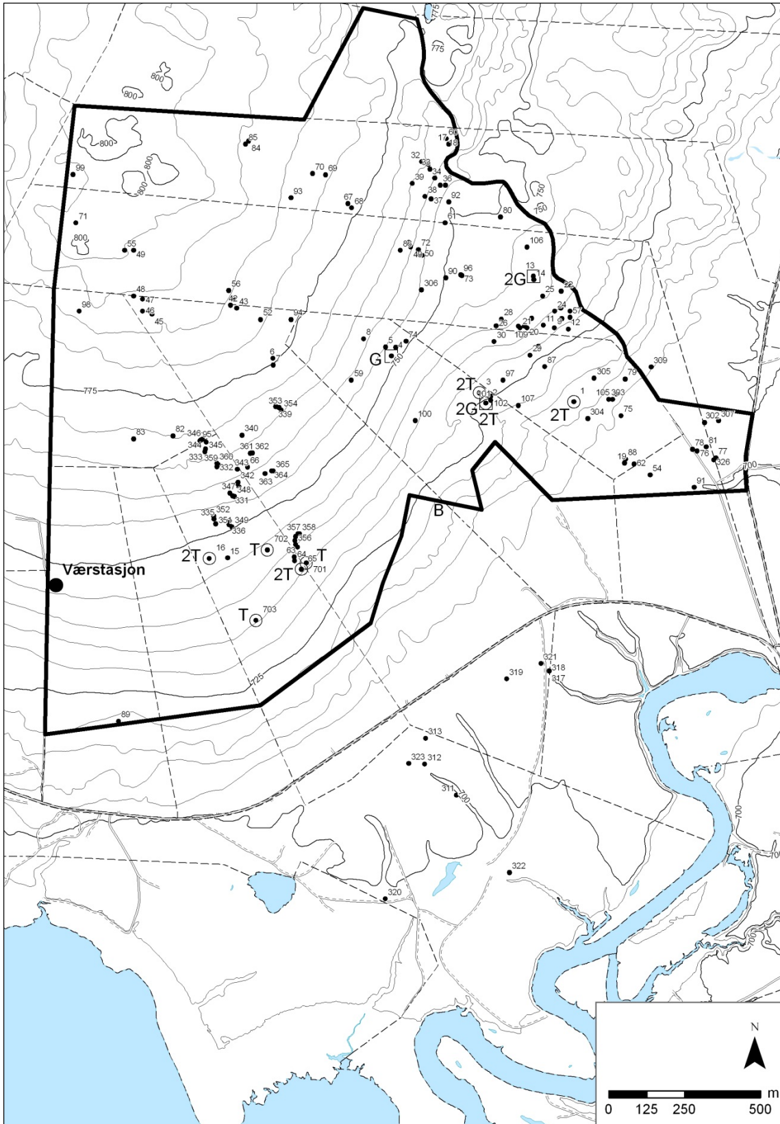
Figur 3. Kart over Sølendet naturreservat som viser plasseringa av 5 grunnvassbrønner (G) for automatisk registrering av vasstandsniå, 13 telemål (T), værstasjon og fastmerka lokalitetar (små nummer). B: Tidlegare beiteområde med fastmerka prøveflater på begge sider av reservatgrensa.
