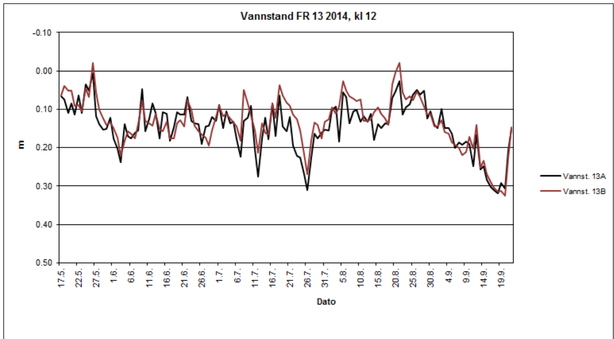
Figur 6. Eksempel på variasjonen i grunnvasstanden gjennom sesongen 2014 på Sølendet. Prøveflate 13A blir slått med ljà i august annakvart år, sist 18. august 2013. Prøveflate 13B har vore uslått sidan 1984.
