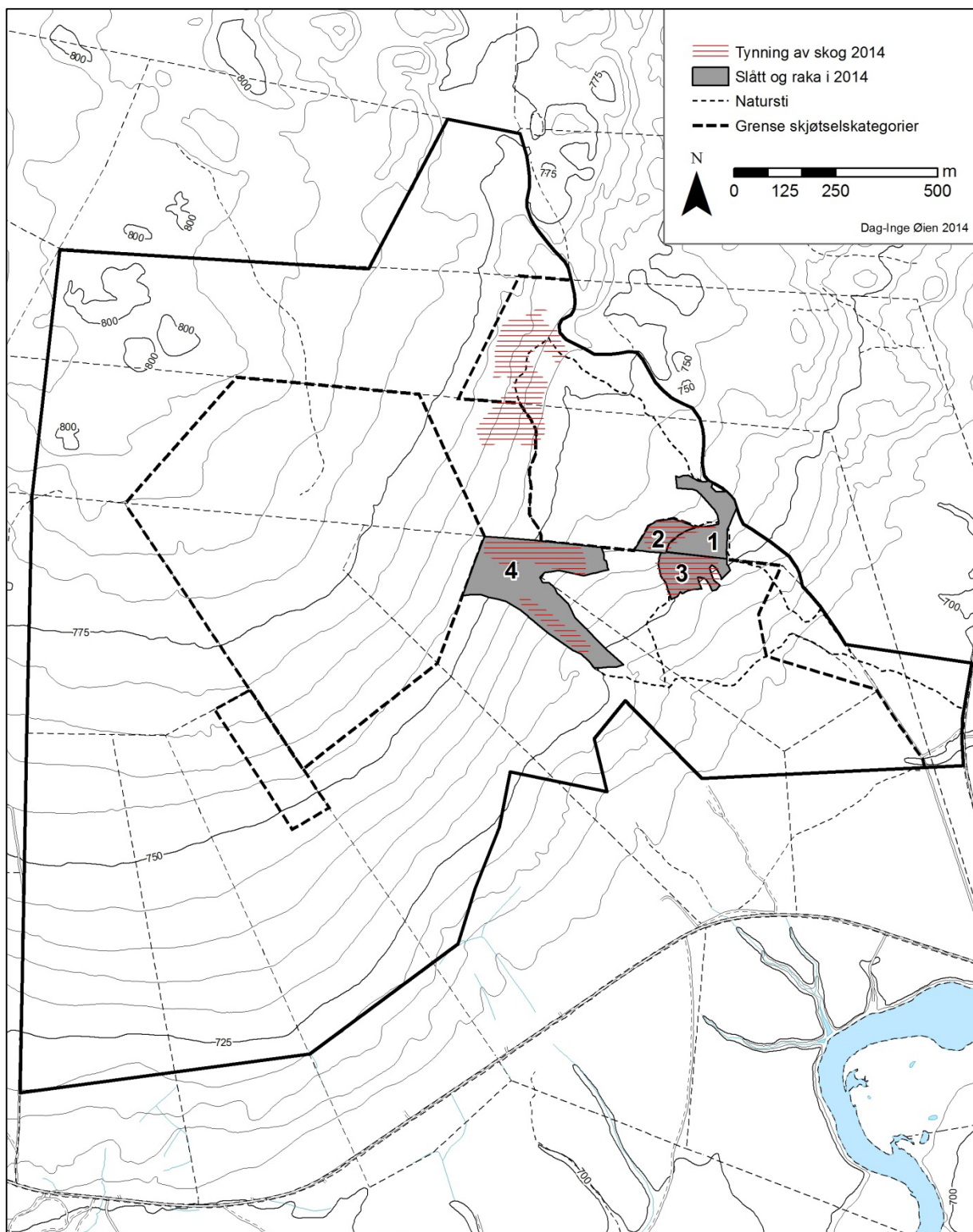
Figur 7. Skjøtta areal på Sølendet i 2014. Slått og raking i alle område. 1: Deler av intensivområdet i aust, 16 daa. 2: Midtliaua V, 7 daa. 3: Olderbuholman, 12 daa. 4: Storesvollen-Klaustrypet, 54 daa. Total vart 89 daa slått, og graset vart raka saman og fjerna innan heile arealet.
