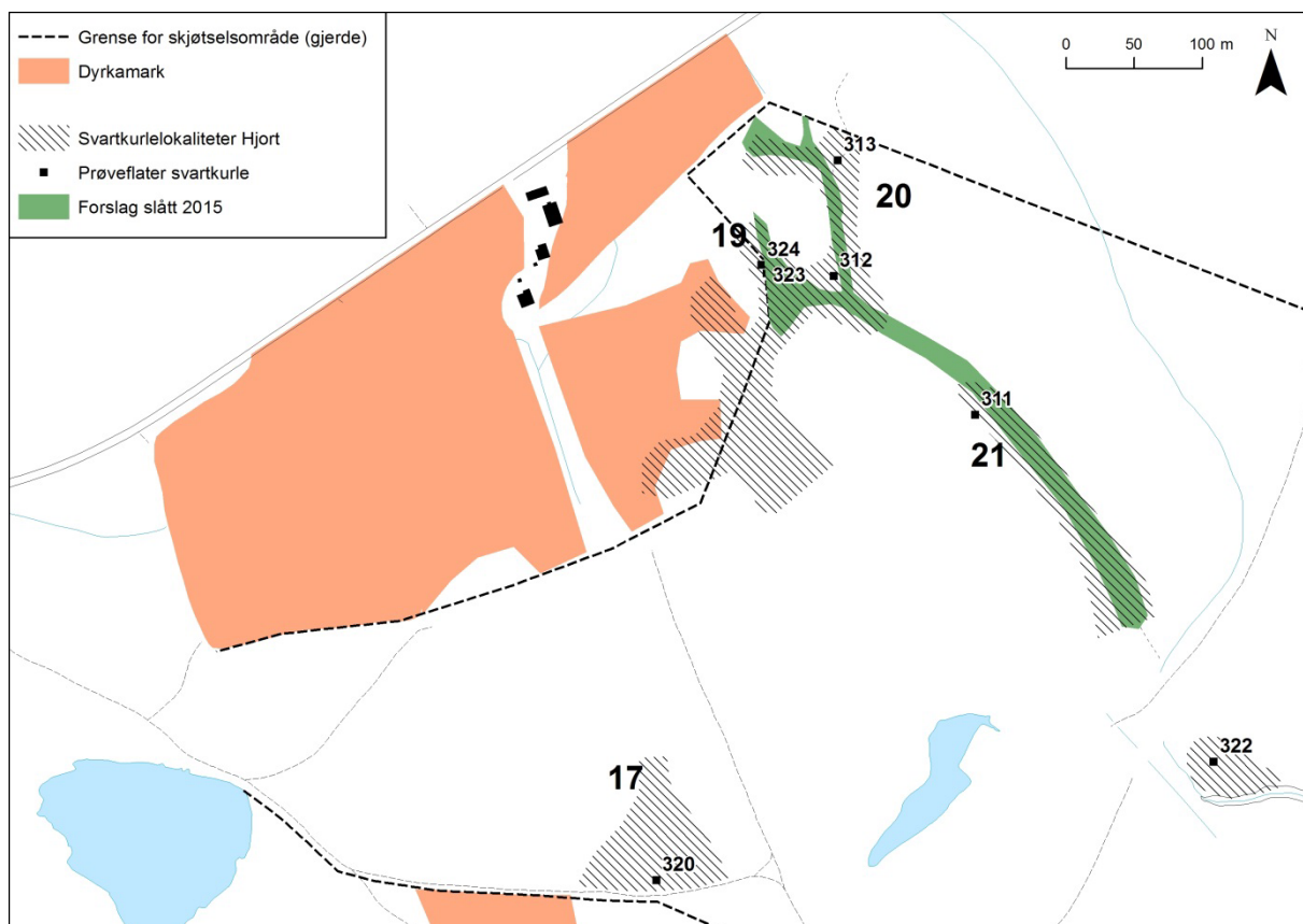
Figur 1. Skjøtselsområdet på Per Hjorts eiendom sør for Sølendet. Plassering av faste prøveflater og angivelse av felt med svartkurle. For 2015 foreslås beiting på samme nivå som før 2013, evt. slått innen område 19-21.
